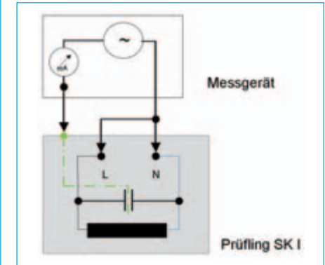
Bild 3-15: Schutzleiterstrommessung im Ersatzableitstrom-Messverfahren bei SK I
