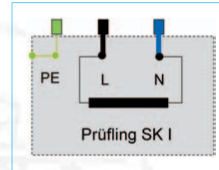
Bild 3-1: Betriebsmittel der Schutzklasse I
