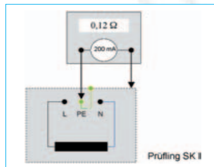
Bild 3-5: Schutzleiterwiderstandsmessung, Prüfling vom Netz getrennt
