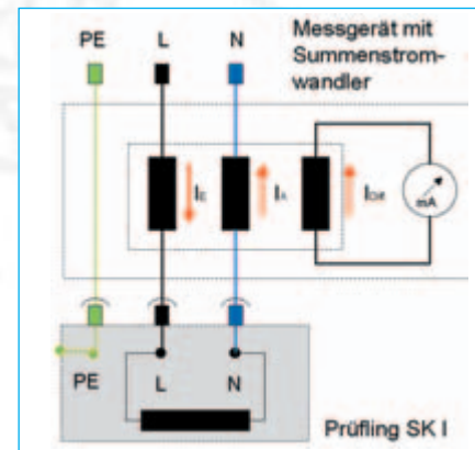
Bild 3-10: Schutzleiterstrommessung nach dem Differenzstromverfahren
