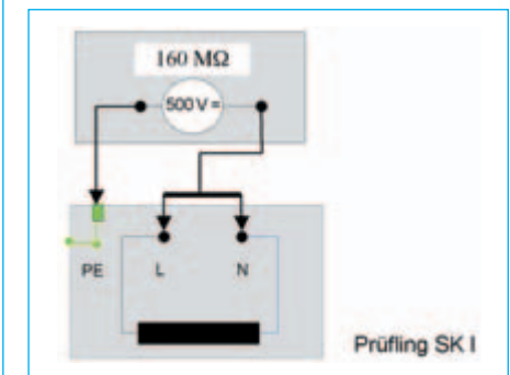
Bild 3-7: Isolationswiderstandsmessung SK I
