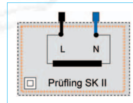
Bild 3-2: Betriebsmittel der Schutzklasse II
