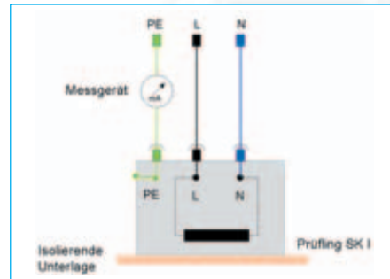
Bild 3-9: Schutzleiterstrommessung als Direktmessung
