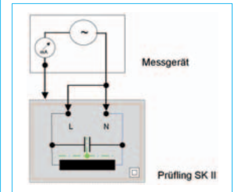
Bild 3-16: Berührungsstrommessung im Ersatzableitstrom-Messverfahren bei SK II
