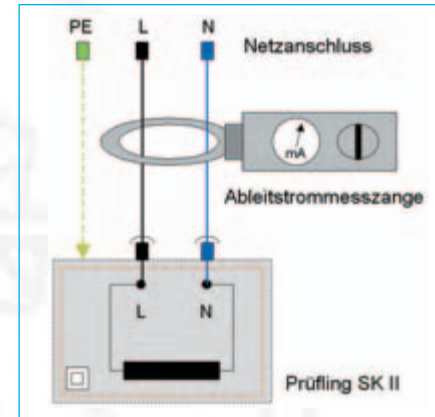
Bild 3-14: Berührungsstrommessung mit einer Ableitstrommesszange (Leckstrommessung) an leitfähigen Teilen, die nicht mit dem Schutzleiter verbunden sind
