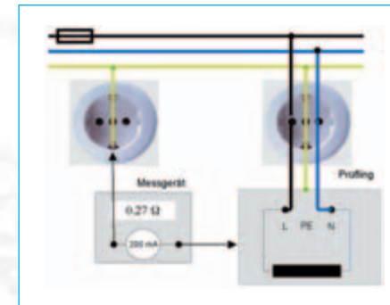
Bild 3-6: Schutzleiterwiderstandsmessung, Prüfling mit Netz verbunden
