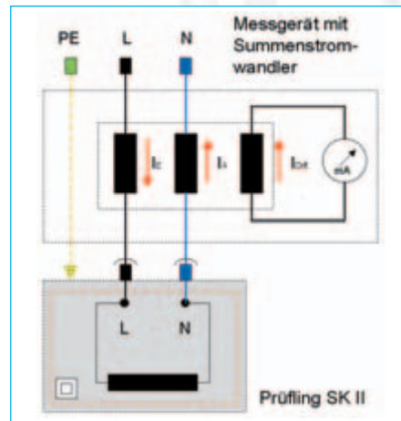
Bild 3-13: Berührungsstrommessung nach dem Differenzstromverfahren an leitfähigen Teilen, die nicht mit dem Schutzleiter verbunden sind
