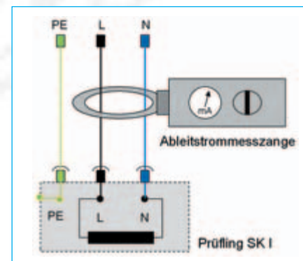
Bild 3-11: Schutzleiterstrommessung mit einer Ableitstrommesszange (Leckstrommessung)
