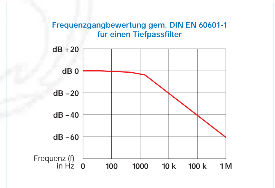
Bild 3-17: Frequenzgangbewertung gemäß DIN EN 60601-1 für die Messanzeige
