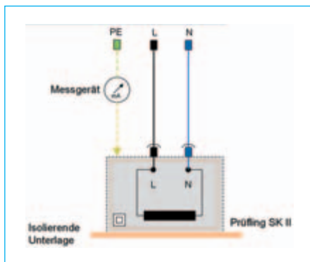
Bild 3-12: Berührungsstrommessung als Direktmessung an leitfähigen Teilen, die nicht mit dem Schutzleiter verbunden sind
