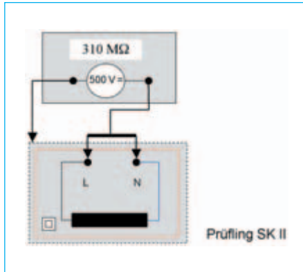
Bild 3-8: Isolationswiderstandsmessung SK II
